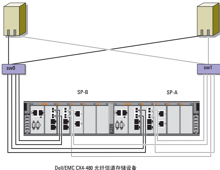
图 2-2. 在 Dell/EMC SAN 连接光纤信道群集中布线
